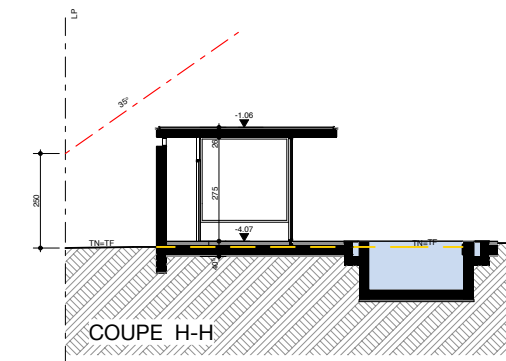
COUPE POOLHOUSE
