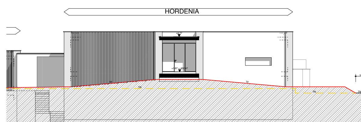
FACADE SUD-EST
