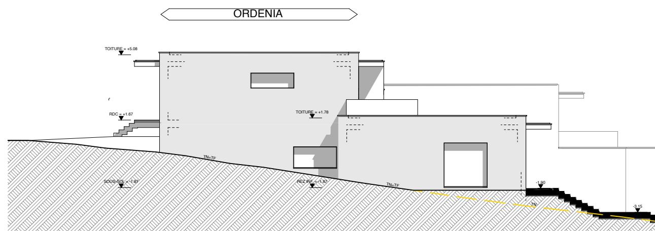
FACADE NORD-EST
