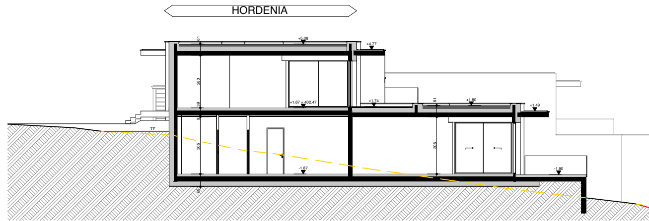
COUPE
